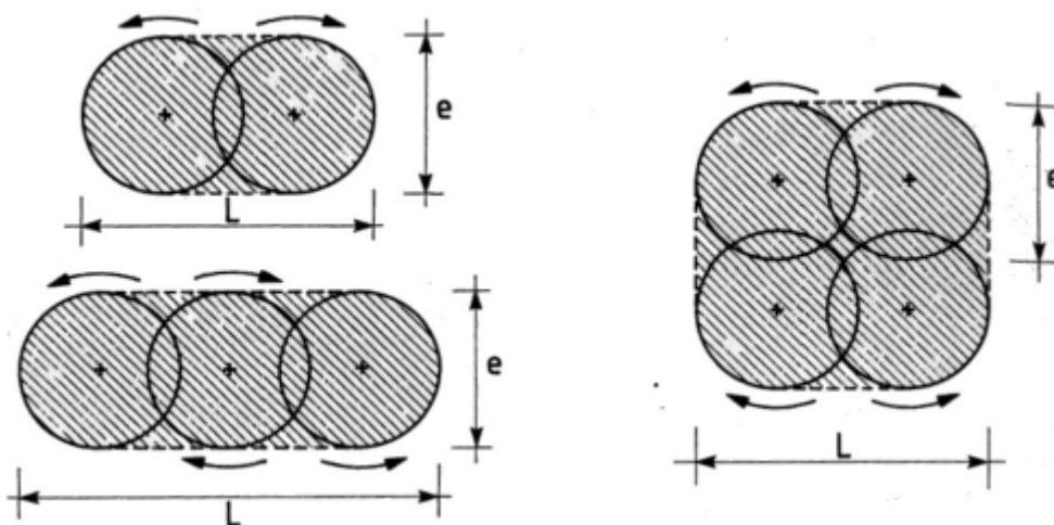
Formes d'une colonne COL MIX
